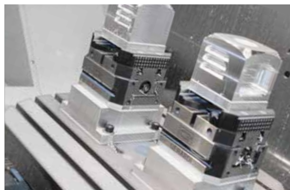
一对虎钳工作时多任务处理 5 轴加工中心的详细信息
