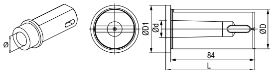
Bloccaggio con grano \ Clamping with set-screw
