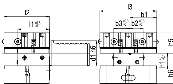
TIPO - TYPE VDI D1 A sedi multiple With multiple seats
