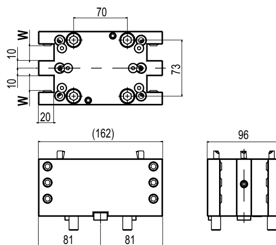
TIPO - TYPE Stelo quadro rad. quadruplo 4 RD face and cutting holder
