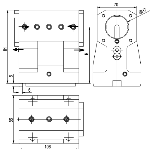
REFRIGERANTE COOLANT Esterno & Interno External & Internal
