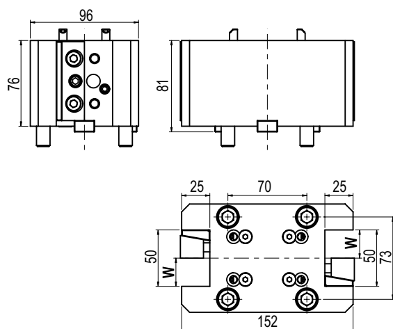
TIPO - TYPE Stelo quadro rad. doppio 2 RD face and cutting holder
