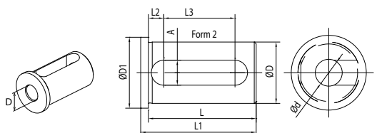
Bloccaggio con asola / Clamping with and slot
