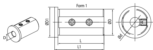
Bloccaggio con asola / Clamping with and slot
