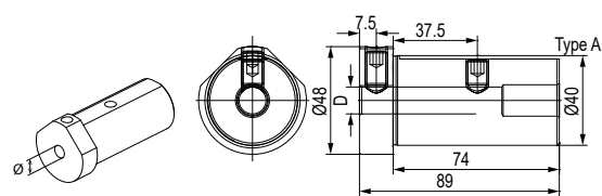
Bloccaggio con grani \ Clamping with set-screws
