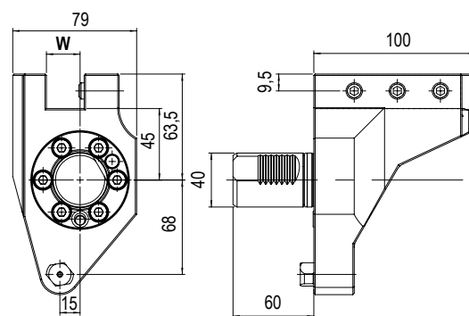
TIPO - TYPE Arretrato Quadro Turning Tool Holder
